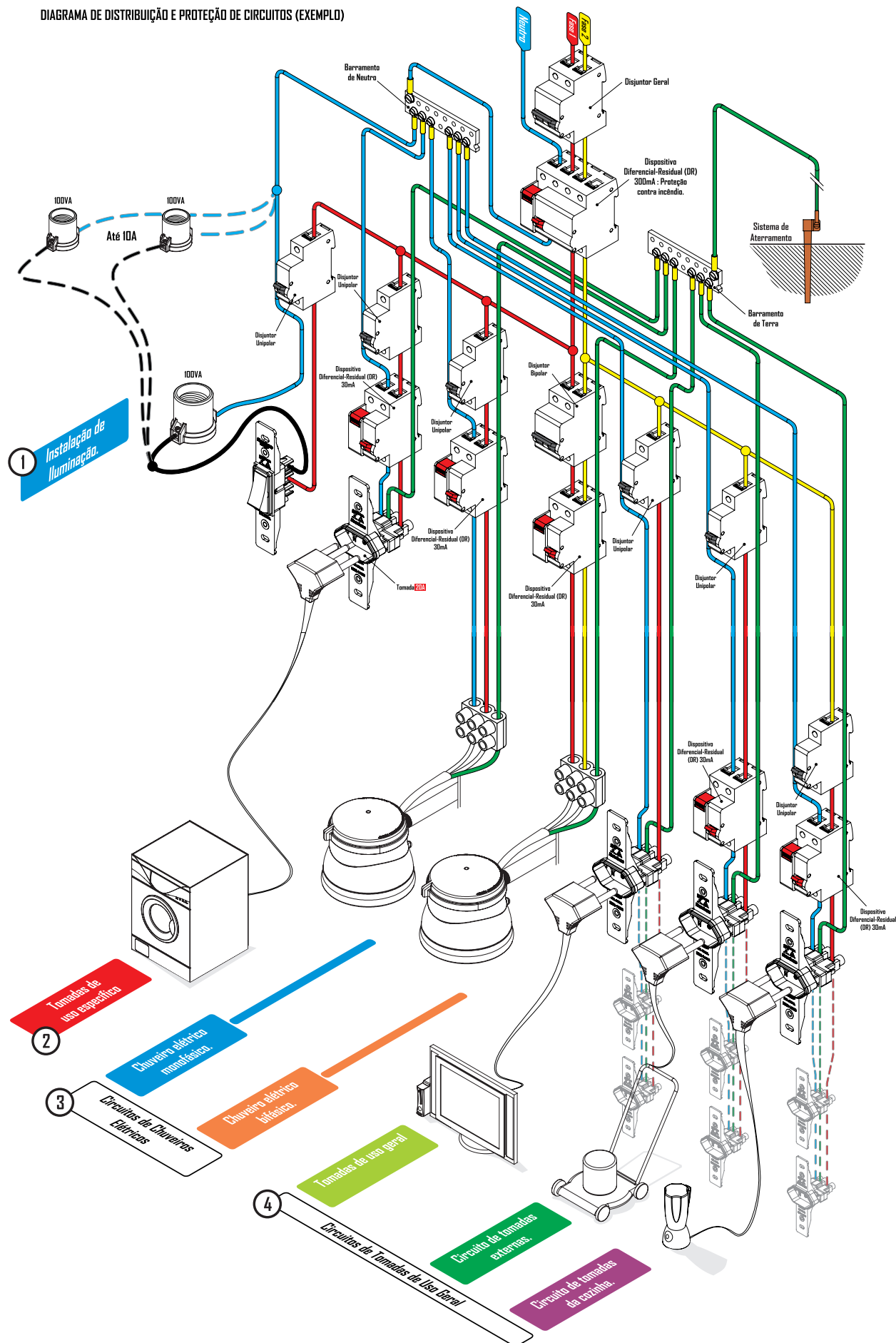
DIAGRAMA DE DISTRIBUIÇÃO E PROTEÇÃO DE CIRCUITOS (EXEMPLO)
