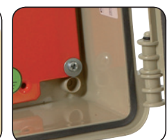
Cavidade para fixar o quadro através de parafusos com tampões de dupla isolamento
